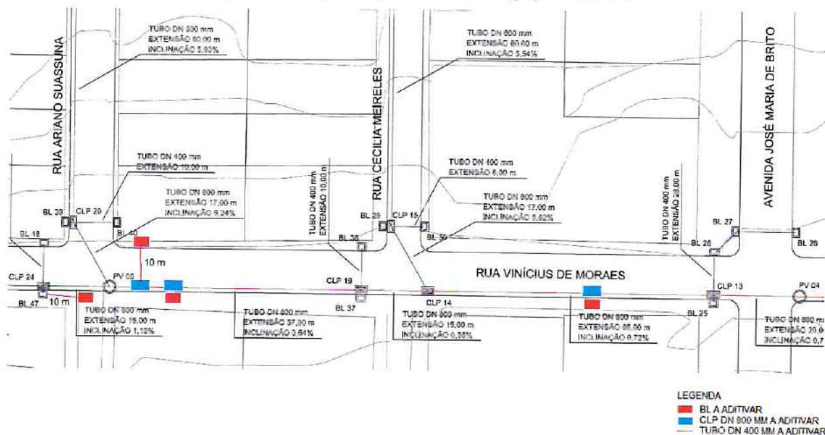
Figura 3 - bocas de lobo e caixas de ligação a aditivar
